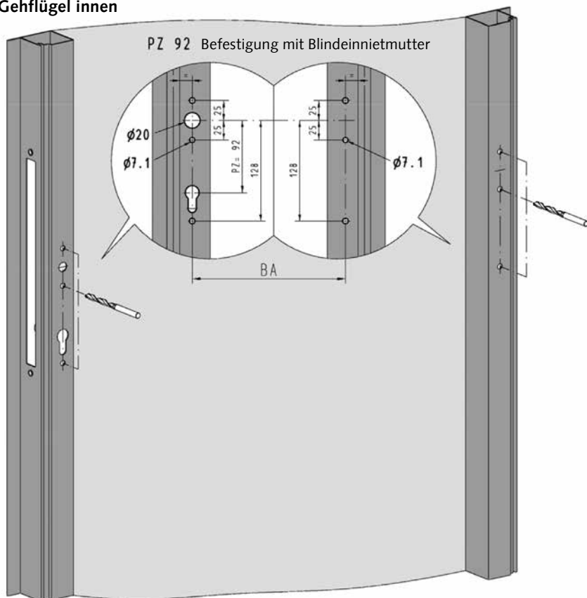
Abb. Gehflügel innen
