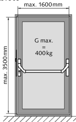
einflügelig – DIN links
