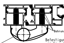
9 Befestigung Tuerband 2-teilig mit Einschraubmuettern
