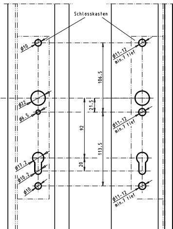
Lochbild Befestigung Schloss
