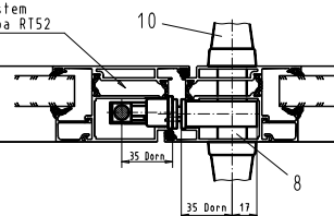
Profilsystem z.B. Alcoa RT52
