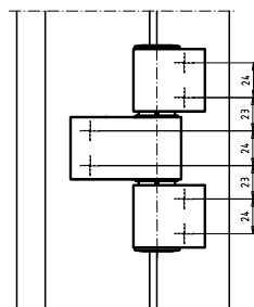
Tuerband 3-teilig
