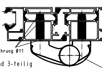
9 Befestigung Tuerband 3-teilig mit Einschraubmuettern
