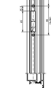
Profilsystem z.B. Alcoa RT52
