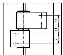
Tuerband 2-teilig
