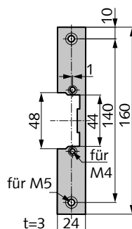
Abbildung Gehflügel DIN links
