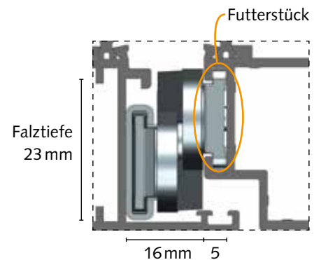
Profilschnitt mit Schere
