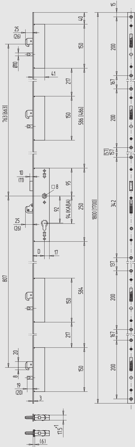
Abbildung DIN rechts, (...) = U-Stulp [...] = Länge 1700 mm
