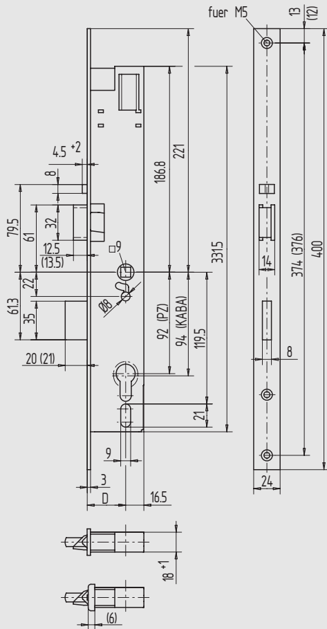
Abbildung DIN rechts (...) = U-Stulp
