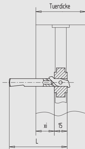
Maßskizze für Spezial-Wechselstift FS 117 für Feuerschutztüren. Türdicke und Maß xi bei Bestellung angeben.
