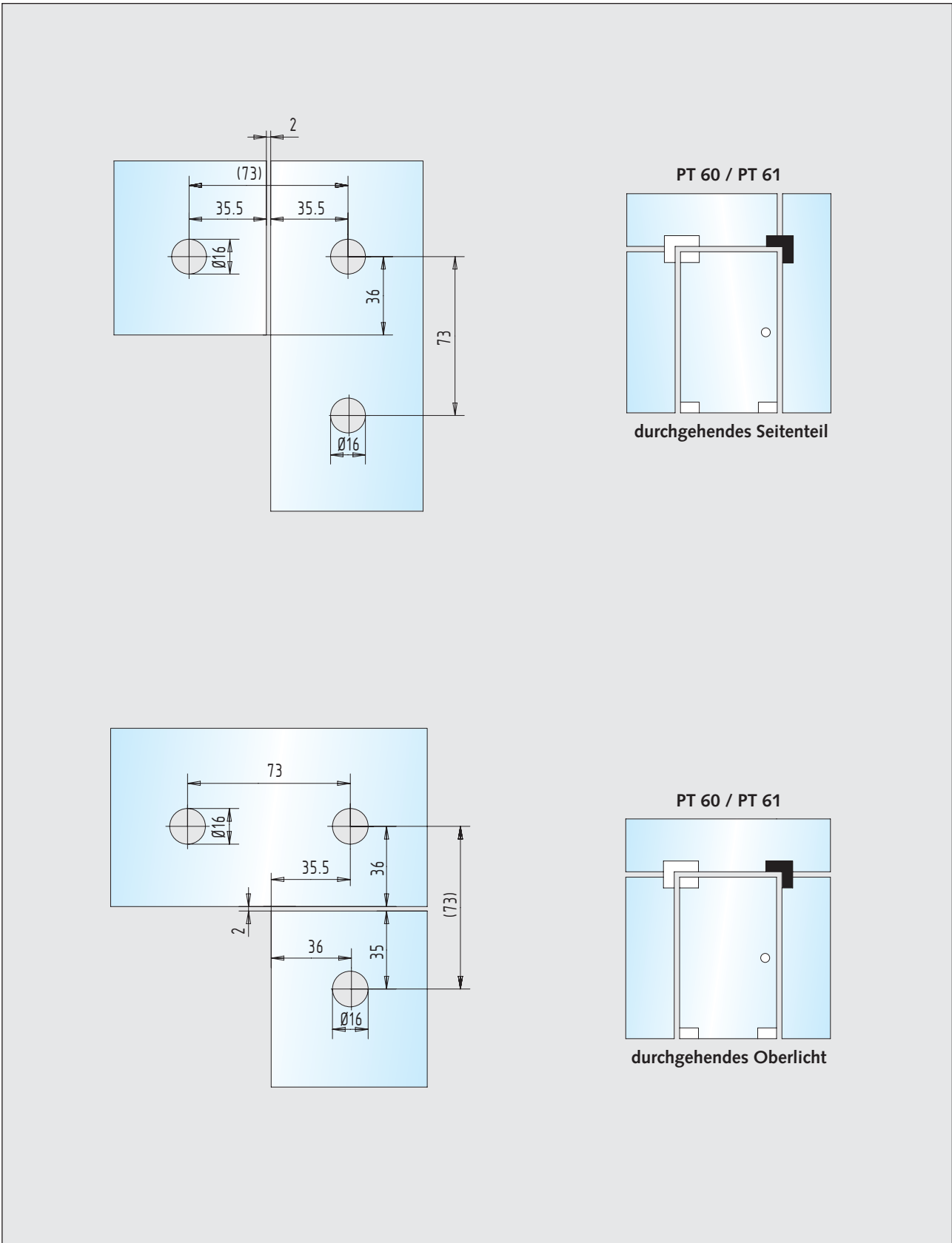
Winkelverbinder
