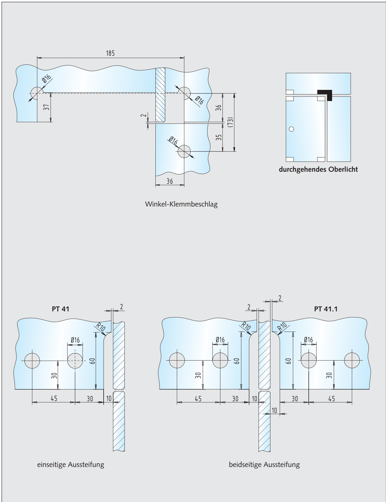
Winkel-Klemmbeschlag / einseitige Aussteifung Winkel-Klemmbeschlag / beidseitige Aussteifung
