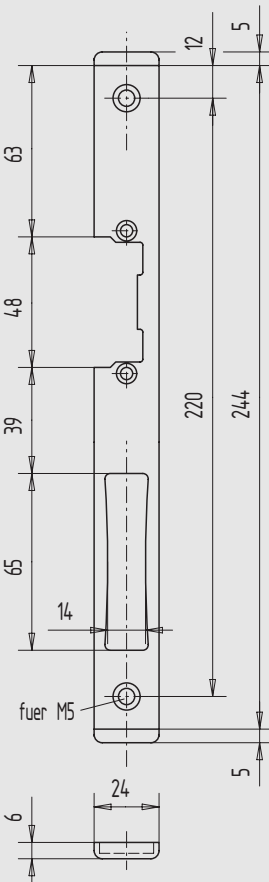
Abbildung für Gehflügel DIN rechts
